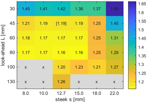
a. genormaliseerde rondetijd T v_0 / L
