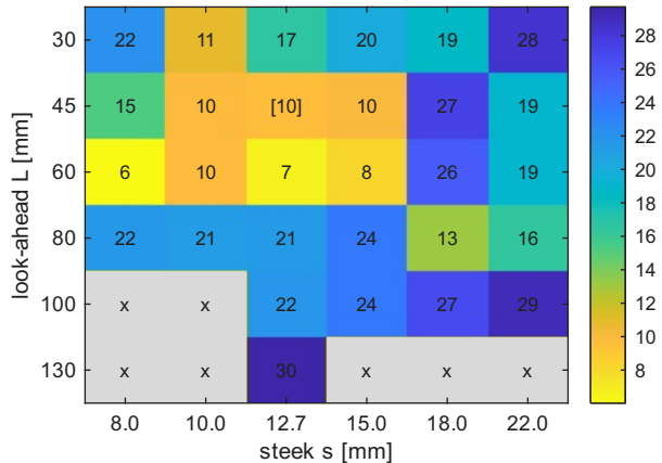
b. grootste afwijking e_{\max} [mm]
